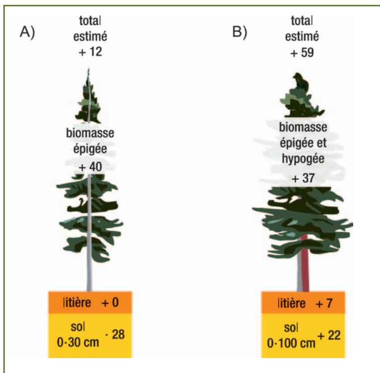
Accumulation du carbone organique (tonnes ha -1 ) estimée au total, dans la biomasse des arbres, la litière et le sol des plantations A) d'épinette blanche et B) de pin rouge sur sol loameux, au cours des 22 premières années.
