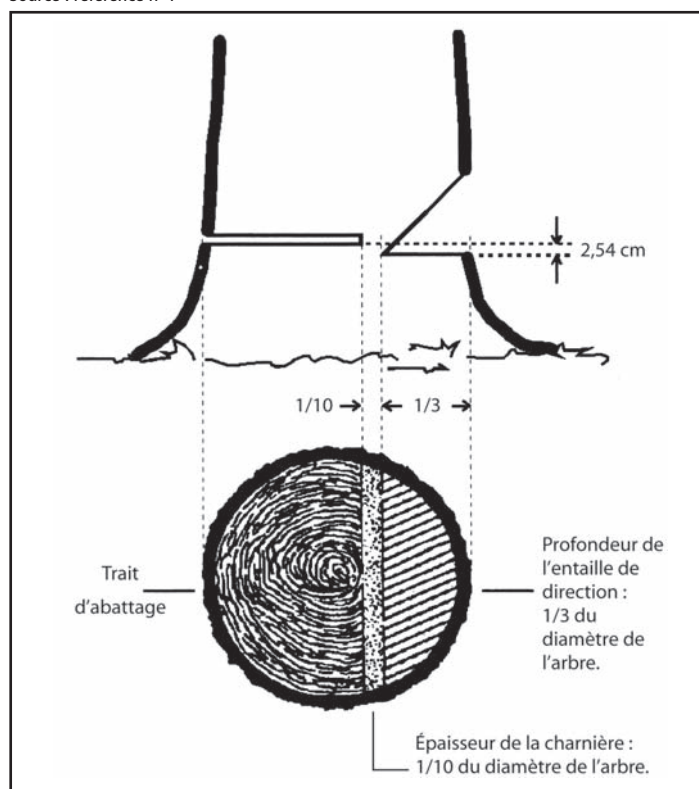
Figure 8 - Réalisation d'une charnière pour le résineux
