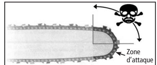
Figure 4 - Forces réactives de la chaîne
